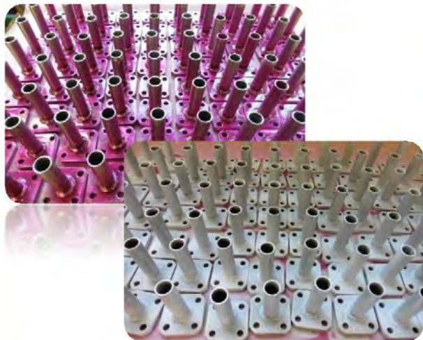
Folyadékbehatolási vizsgálat
